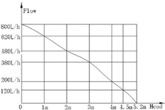
特性曲线图
